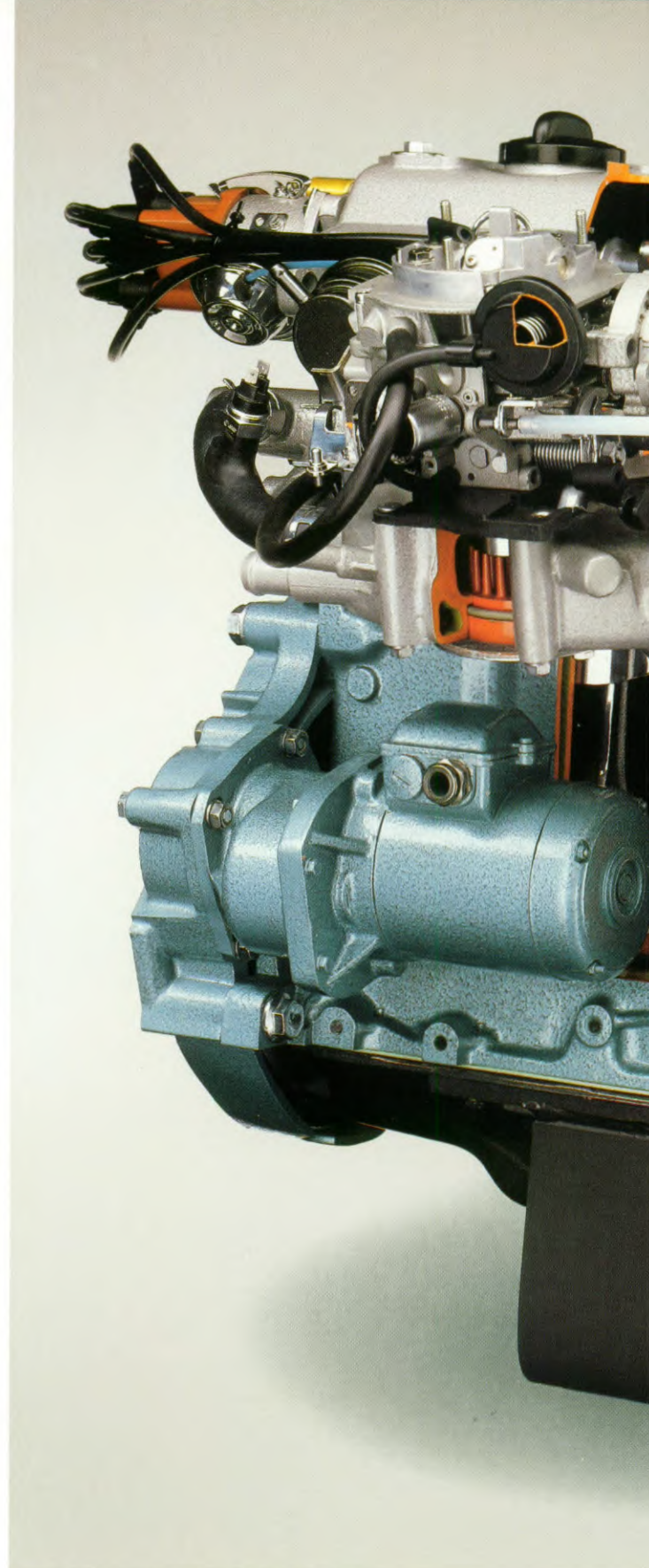
Opengewerkt model van de 40 kW (55 pk) motor
