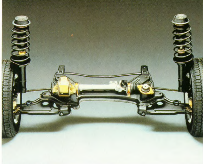
Voorwielophanging
