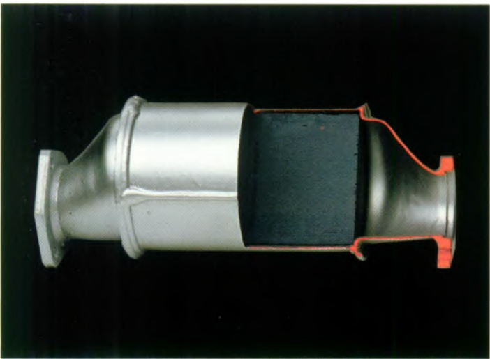
De katalysator. De katalysator maakt milieuvriendelijk autorijden mogelijk. Hij vermindert de uitwerping van schadelijke bestanddelen in het uitlaatgas en is dankzij de lambda-regeling uitermate effectief.
