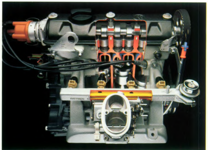
De Digijet-motor (niet leverbaar in Nederland). Deze elektronisch gestuurde injectie-motor is bijzonder "schoon" door zijn katalysator met lambda-regeling. Bijzonder kenmerk is een hoog koppel bij lage toerentallen.
