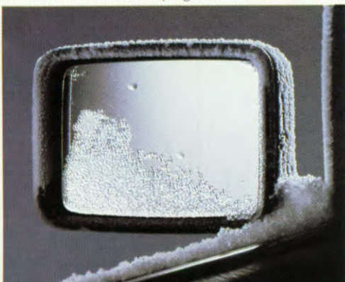
De verwarmbare buitenspiegel.
