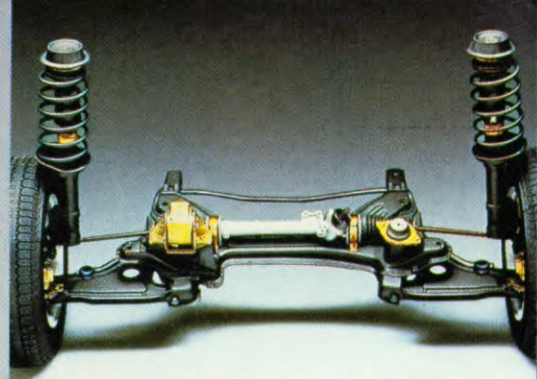
De vooras met zelfcorrigerende stuurinrichting.
