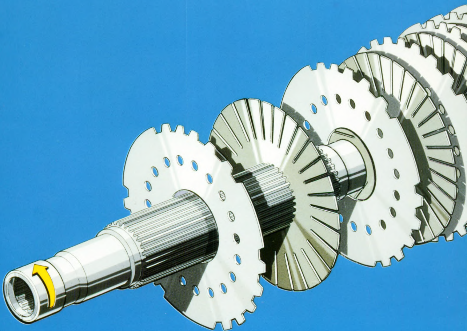
De stalen lamellen van de visco-koppeling.
