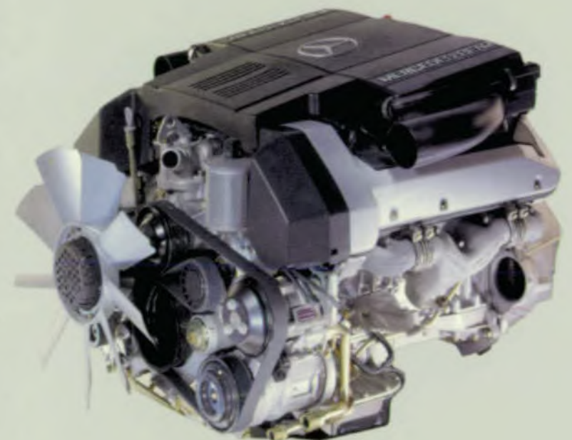
De achtcilinder motor met 32 kleppen.
