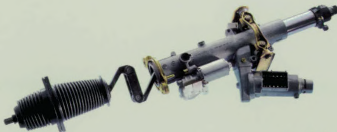
De elektrisch verstelbare stuurkolom. Met één druk op de knop de ideale stand.
