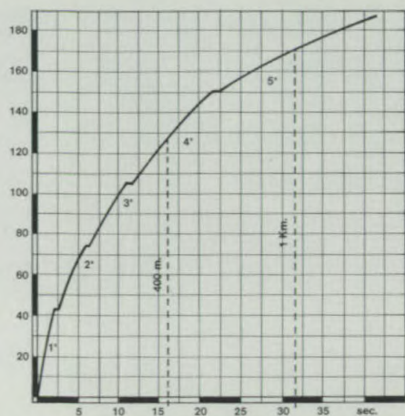
acceleratiecurve
