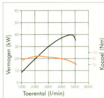
Vermogen en koppel van de 1,6 liter dieselmotor.
