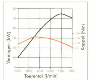
Vermogen en koppel van de 1,6 liter benzine-motor.
