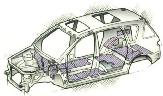
De carrosserie heeft een hoge torsiestijfheid. Tezamen met het dempingsmateriaal op strategische punten zorgt dit voor een aangenaam stil interieur.
