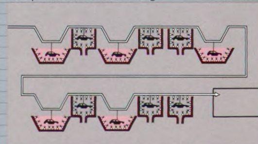
Elektrostatische lakbehandeling
