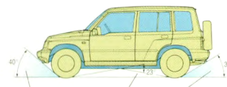
Inloophoek, Bodemvrijheid, Uitloophoek
