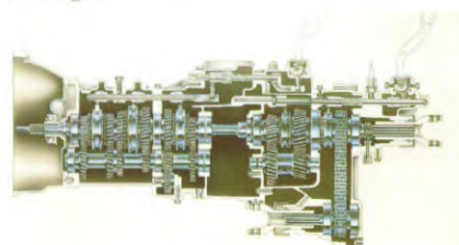
de transmissie en de tussenbak staan in elkaars verlengde
