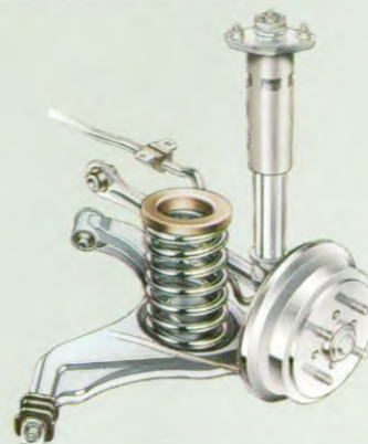
Onafhankelijke achterwielophanging
