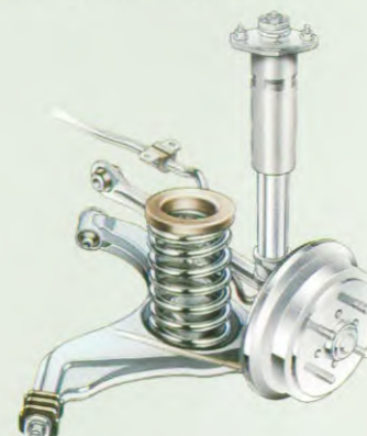
Onafhankelijke achterwielophanging
