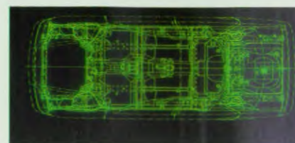
Computer Aided Design (CAD) voor minimaal gewicht en maximale stijfheid
