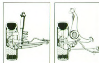
Onafhankelijke wielophanging.
