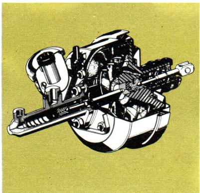
Mastervac rembekrachtiging, waardoor de benodigde druk op het rempedaal aanzienlijk wordt verminderd.
