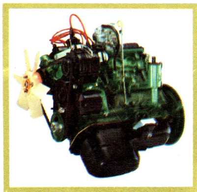
Benzinemotor XC7 - Overvierkante 4 cilinder lijnmotor 45° gekanteld - Boring x slag 84 x 73 - Cilinderinhoud : 1.618 cc.
