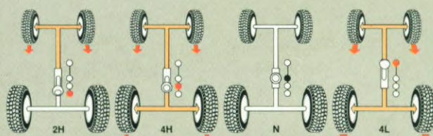
5-bak, voorwielaandrijving in- en uitschakelbaar via tussenbak met hoge en lage gearing.
