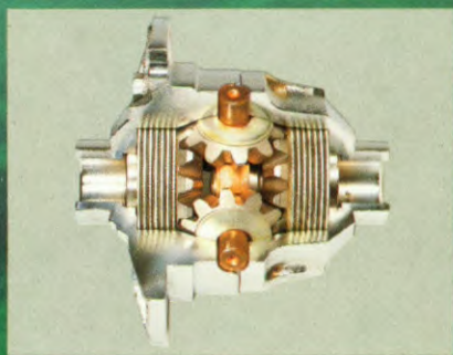
Limited-slip differentieel.
