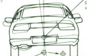
Oorspronkelijke rolas Gecontroleerde rolas bij overhellen
