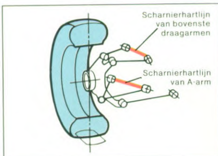
Draaihartlijn van de carrosserie bij het ontbreken van lift- en duikkrachten
