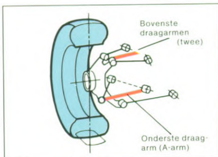
Dynamische controle van de rolhartlijn (bij het sturen naar rechts)
