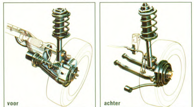
Wielophanging voor en achter onafhankelijk (Wagon achter: torsie-as).
