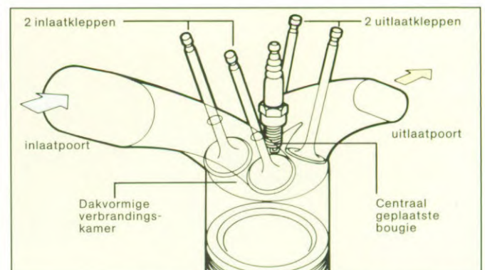
Door toepassing van multi-kleppen techniek "ademt" de benzinemotor gemakkelijker. Door deze drastische rendementsverhoging presteert de Sunny méér met minder brandstof.
