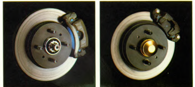
Geventileerde schijfremmen vóór zorgen voor betere koeling en optimale remkracht. (GTi: schijfremmen rondom).
