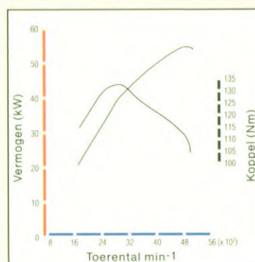
CD20 2.0 liter dieselmotor. Maximaal vermogen 55/4800 kW/tpm; maximaal koppel 132/2800 Nm/tpm.
