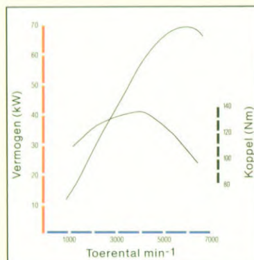
GA16DS prestatie motor, 1.6 liter. Maximaal vermogen 66/6000 kW/tpm; maximaal koppel 133/4000 Nm/tpm.
