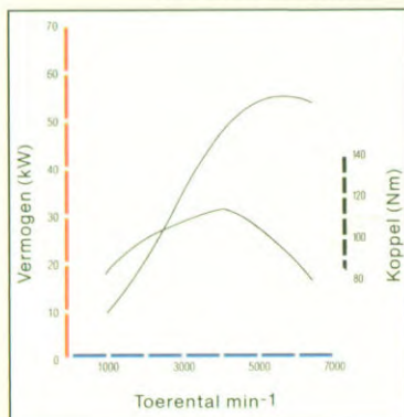
GA14DS superzuinige motor van 1.4 liter. Maximaal vermogen 55/6000 kW/tpm; maximaal koppel 112/4000 Nm/tpm.
