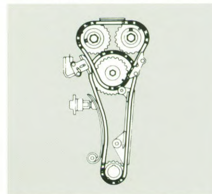
Onderhoudsvrije nokkenasbediening
