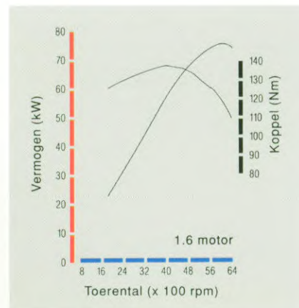
Vermogens- en koppelkromme
