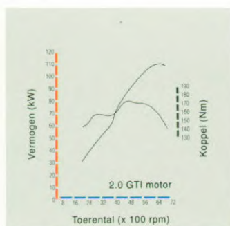
Vermogens- en koppelkromme
