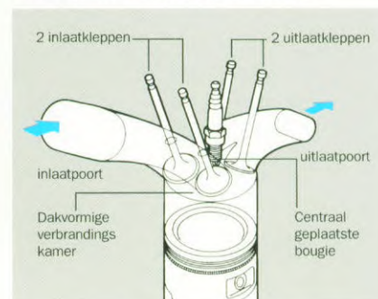
Dakvormige verbrandingskamers met centraal geplaatste bougies.
