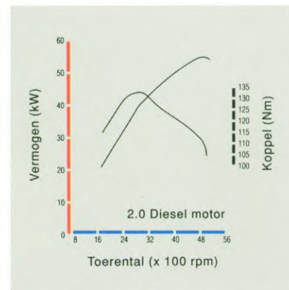
Vermogens- en koppelkromme
