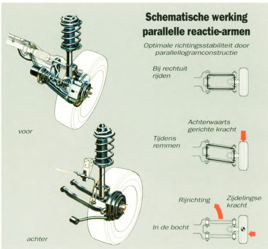
Uitgebalanceerde wielophanging
