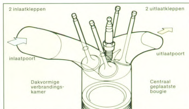
Door toepassing van multi-kleppen techniek "ademt" de benzinemotor gemakkelijker. Door deze drastische rendementsverhoging presteert de Sunny méér met minder brandstof.
