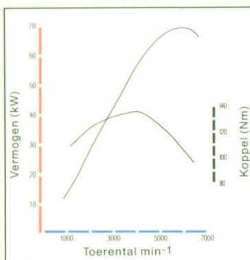
GA16DS prestatie motor, 1.6 liter. Maximaal vermogen 66/6000 kW/tpm; maximaal koppel 133/4000 Nm/tpm.
