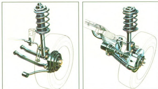
Wielophanging voor en achter onafhankelijk (Wagon achter: torsie-as).
