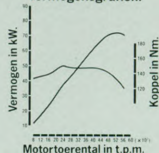
Vermogensgrafiek.
