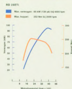
Vermogens- en koppelkromme 2,8 liter 6-cilinder Turbo diesel intercooler.
