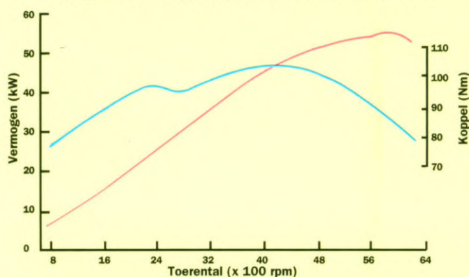
Vermogens- en koppelkromme van de 1.3 motor.
