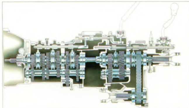
Dwarsdoorsnede van de versnellingsbak en de tussenbak
