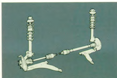
Onafhankelijke wielophanging vóór. Achterasconstructie met vier reactie-armen.
