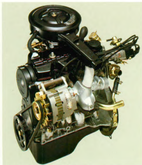
Lichte compacte motor...
