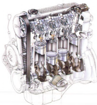
1.6-liter, 16-kleppenmotor.
