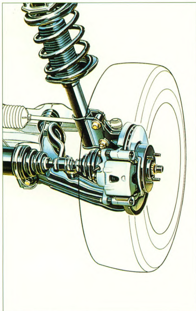
Mc. Pherson voorwielophanging
