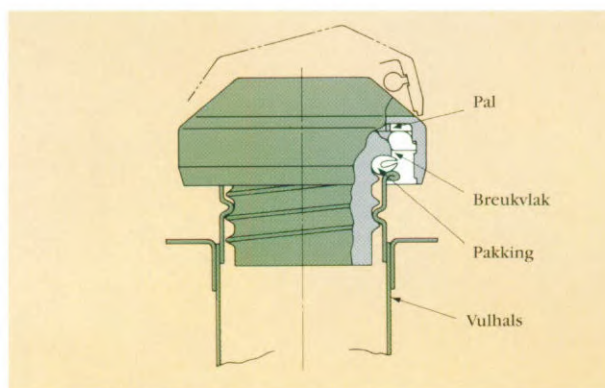
Een speciale schroefdoop verkleint het gevaar op brand.
