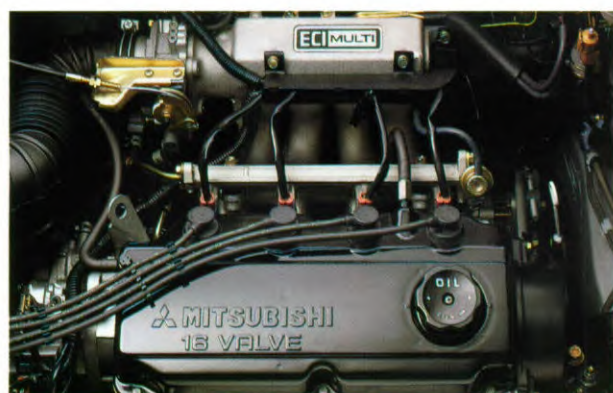
De 1.8 liter SOHC 16 kleppen motor met ECI-MULTI
