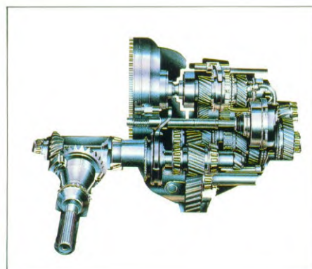
4WD transmissie.
