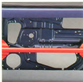
Stalen stangen in de portieren bieden bescherming bij frontale en zijwaartse aanrijdingen.
