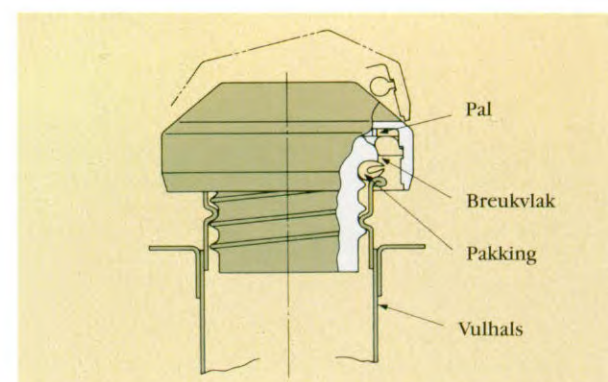
Een speciale schroefdoop zorgt voor een betere afdichting en voorkomt lekkage bij het tanken.
