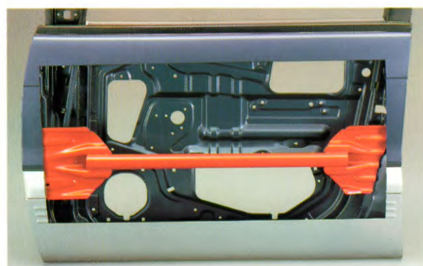
Stalen profielen in de portieren bieden bescherming bij frontale en zijwaartse botsingen.
