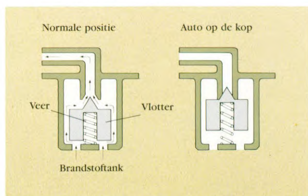
Een speciale afsluitklep in de tank voorkomt lekkage in geval van een ongeval.
