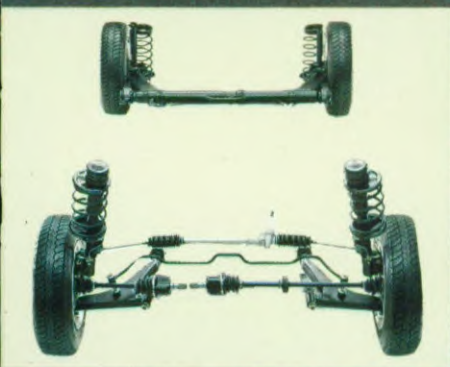
Rondom onafhankelijke wielophanging McPherson veerpoten met excentrische spiraalveren, stabilisatorstang vóór en achter, en deU-vormige achteras met progressieve veren
