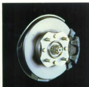
MacPherson onafhankelijke voorwielophanging met schroefveren en stabilisator
