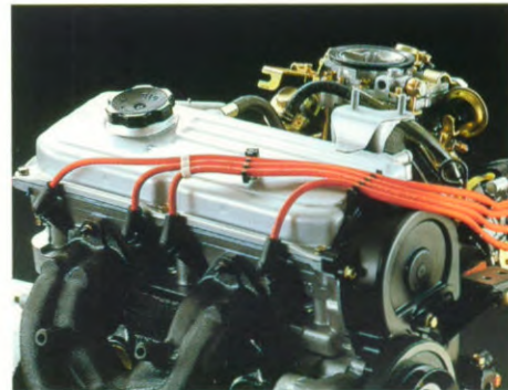
1,5 liter benzinemotor (Vermogen 55 Kw/5500 rpm.)
