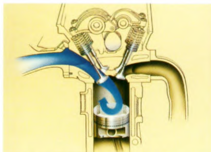
Door de bijzondere vorm van de verbrandingskamers en de centraal geplaatste bougies wordt een optimale verbranding en een krachtiger vermogen verkregen.
