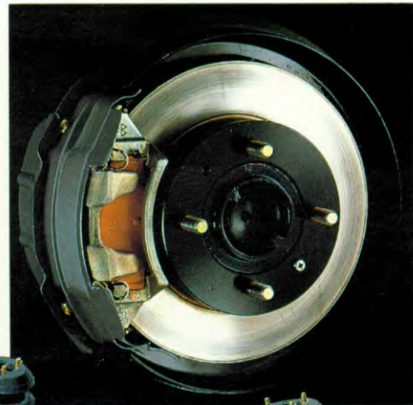
Schijfremmen achter (GLS modellen).
