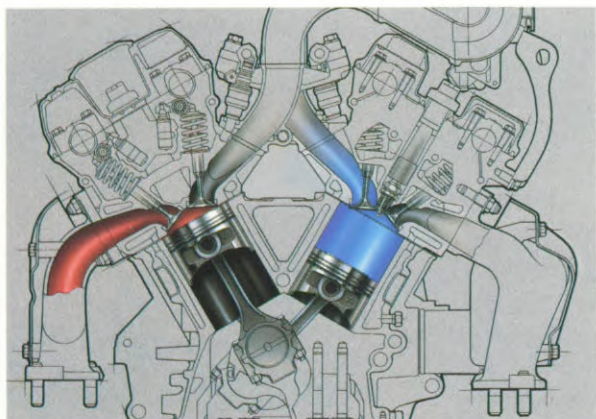
Zowel de V6 DOHC 2.0 liter als de 2.5 liter motor zijn uitgerust met luifelvormige verbrandingskamers. Dat betekent extra motorrendement en een krachtig en soepel vermogen.
