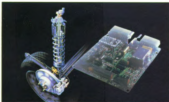
MacPherson voorvering met extra rubber damping voor geluid en trillingen.
