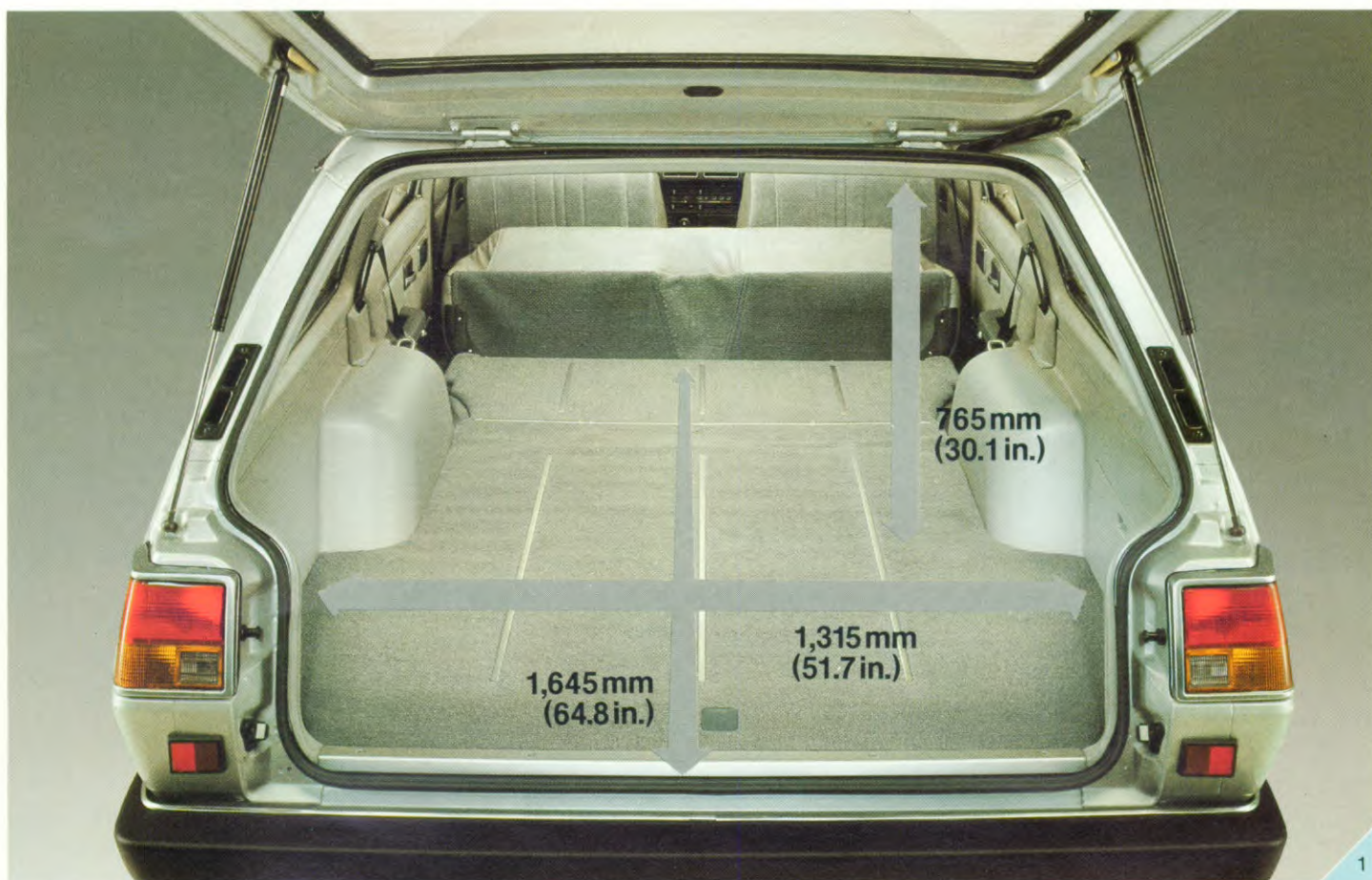
De ruim bemeten, vlakke laadvloer van de Galant Stationwagon is dankzij de grote achterklep goed te bereiken. De van gasgevulde dempers voorziene achterklep scharniert hoog op, wat in- en uitladen vergemakkelijkt.
