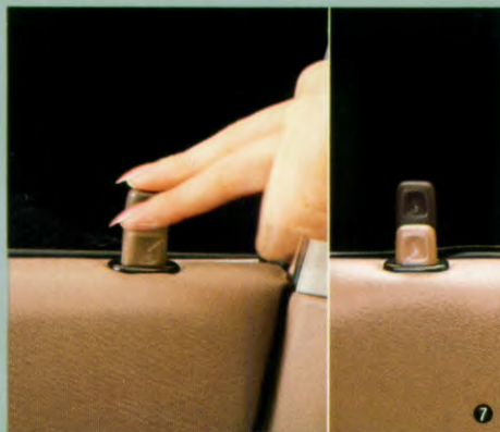
Centrale deurvergrendeling,
