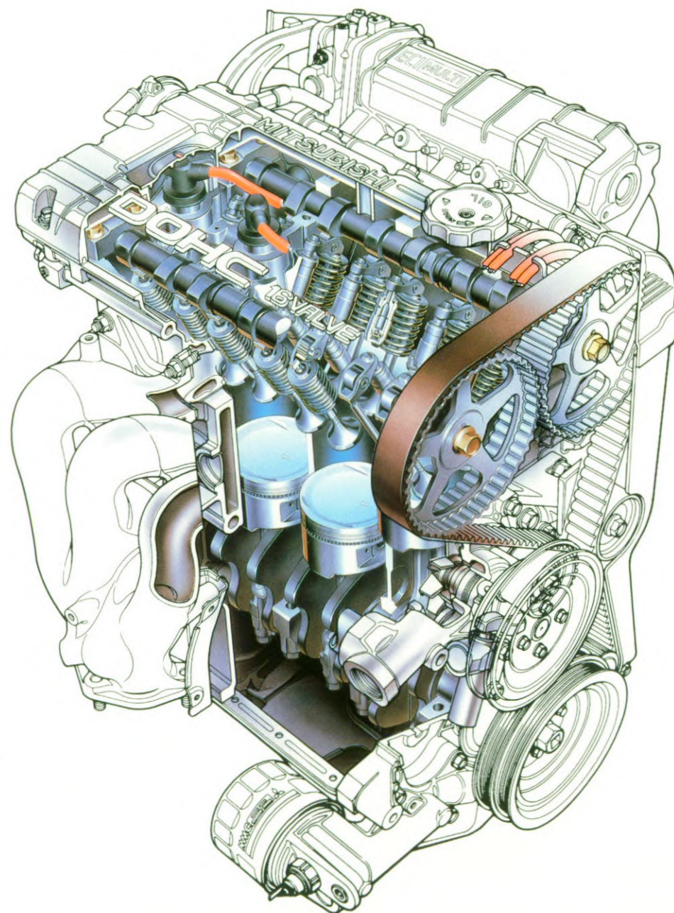
16-kleppen ECI-Multi motor (1.6 GTi-16V) - Maximum snelheid: 195 km/h - Maximum vermogen: 91 kW/6500 tpm - Maximum koppel: 142 Nm/5000 tpm
