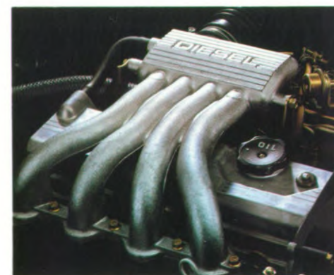
Dieselmotor (Colt diesel niet leverbaar in Nederland).
