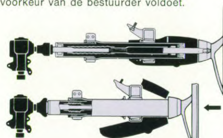
Schokabsorberende stuurkolom
