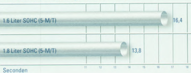
Acceleratie in 5de versnelling (80 km/h tot 120 km/h)
