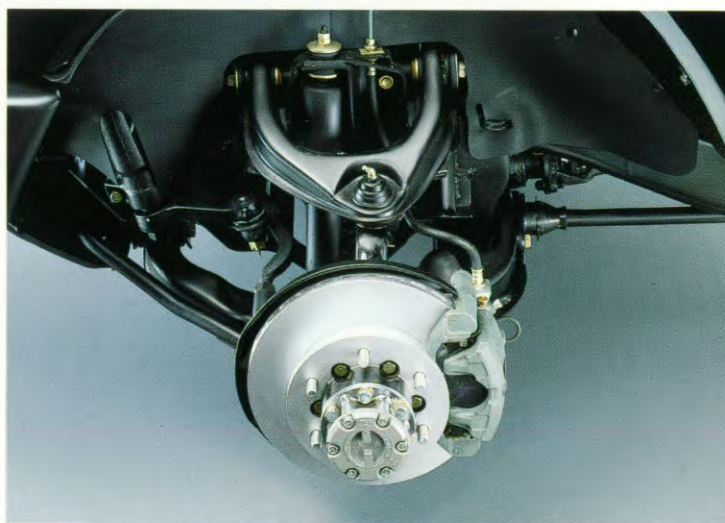
Onafhankelijke voorwielophanging met wishbone en torsiestang, en geventileerde schijfremmen.
