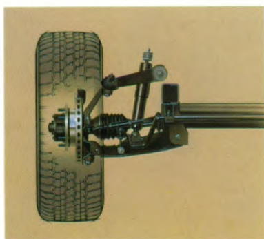
De onafhankelijke voorwielloophanging met dubbele draagarmen en een torsiestang zorgt op elke ondergrond voor een comfortabel en voorspelbaar rij- en stuurgedrag.
