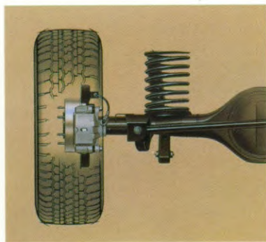
De achterwielloophanging wordt gevormd door de driehoeks reactie-arm in combinatie met schroefveren. Hierdoor krijgt de Pajero gelijkmatige en controleerbare eigenschappen.
