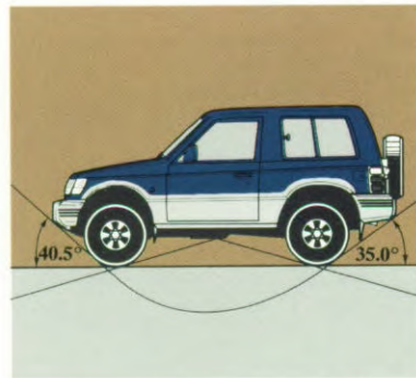
Door de gunstige inrijhoek, de ideale hellingshoek en het enorme klimvermogen is de Pajero onbegrensd in zijn mogelijkheden. Op elk terrein, op elke ondergrond bepaalt u de richting.
