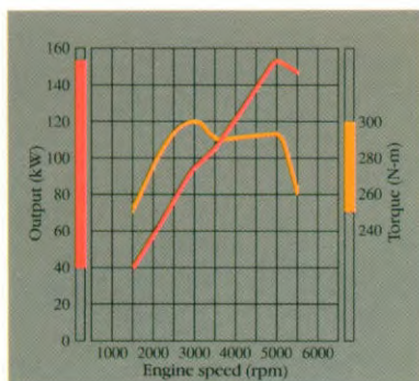
Veel vermogen bij hoge en lage toeren is kenmerkend voor de 3.5 liter V6-24.
