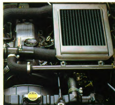
De 2.5 liter turbo dieselmotor intercooler is voorzien van een aluminium cilinderkop.
