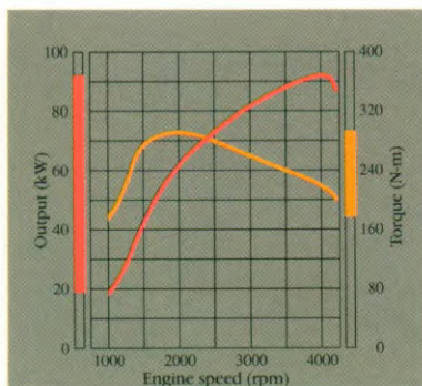
De economische en tegelijkertijd felle 2.8 liter SOHC turbo diesel intercooler levert veel vermogen bij lage toerentallen.
