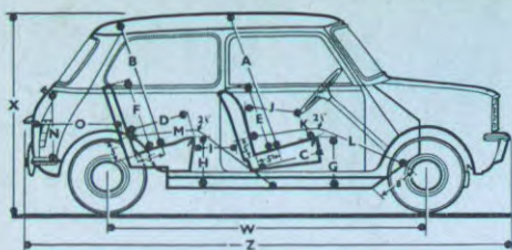
AFMETINGEN CLUBMAN SALOON
