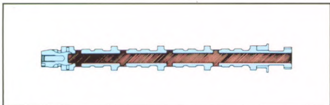
Holle nokkenas
