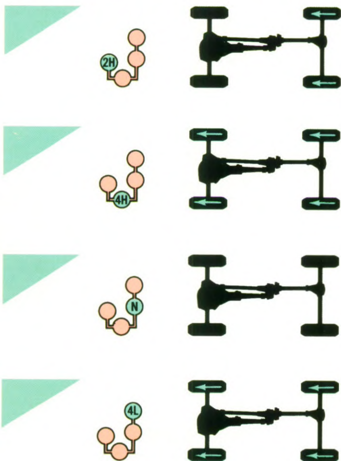
Inschakelbare vierwielaandrijving
