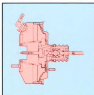
Rembekrachtiging standaard op SJ 413 uitvoering
