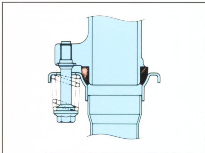
Flexibele veerbevestiging van de uitlaat
