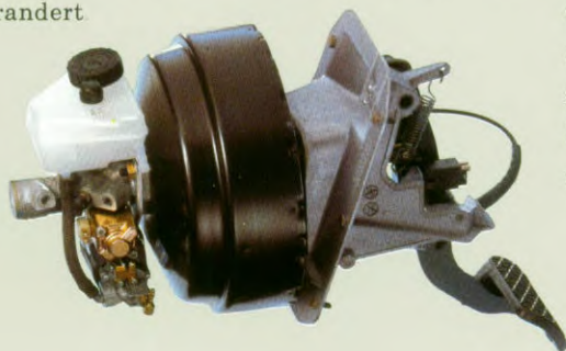
De hoofdremscilinder met rembekrachtiger van de nieuwe S-klasse.
