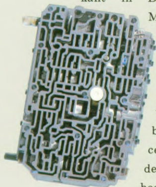
Het hydraulische regelhuis is het "brein" van een automatische versnellingsbak.
