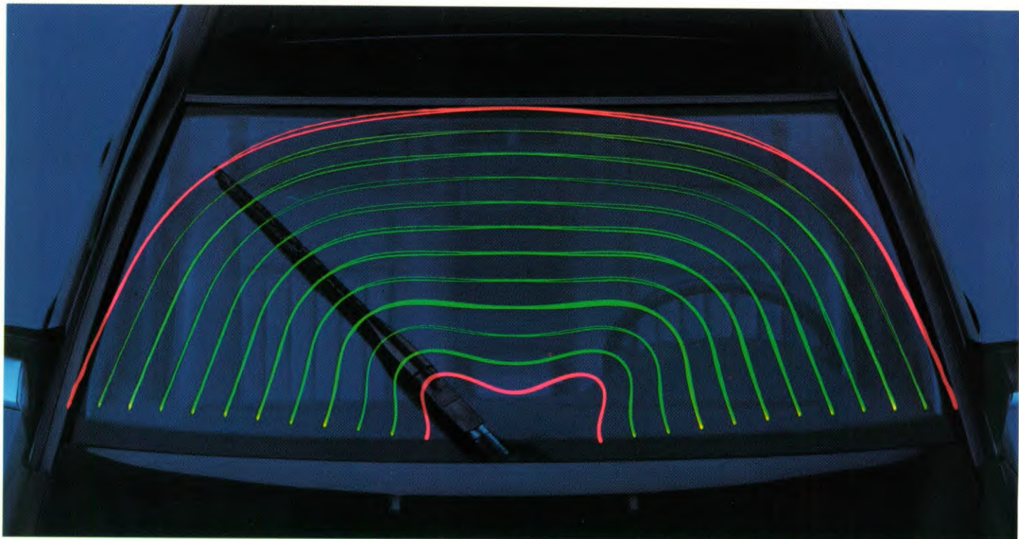
De Panorama-ruitewisser houdt 86% van de voorruit schoon – het maximum dat haalbaar is in de huidige automobiellbouw.
