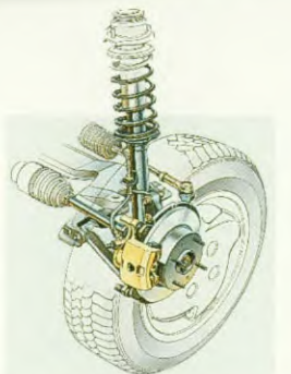
MacPherson-veerpoten vóór en forse schijfremmen zorgen in de Subaru Vivio voor ongekende rij- en remeigenschappen.
