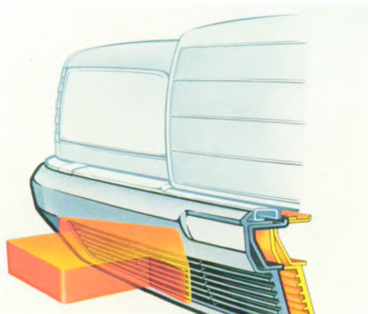
Flexibele bumpers vangen schokken tot 4 km/uur op zonder kans op schade.
