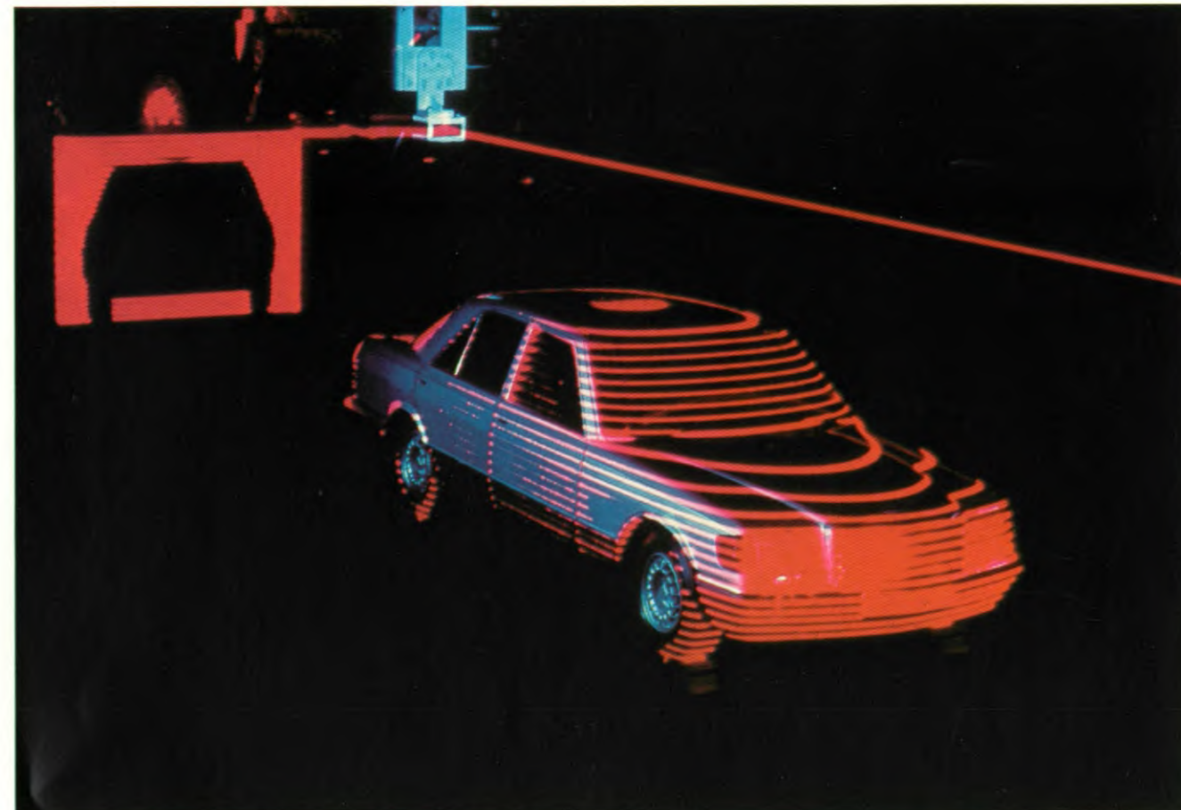
Door afmeting met een laserstraal wordt het frontoppervlak bepaald, tot op de millimeter nauwkeurig.
